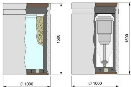
Schémas de conteneurs amiante-ciment
